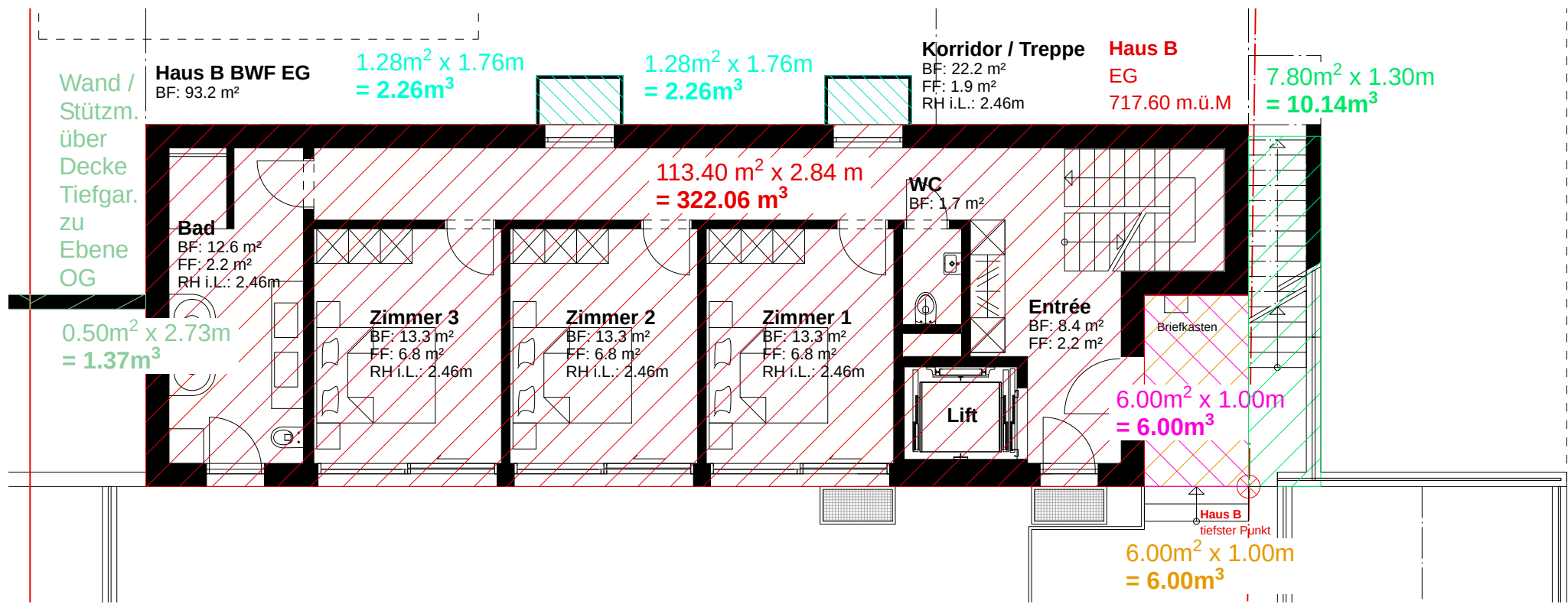
Erdgeschoss
