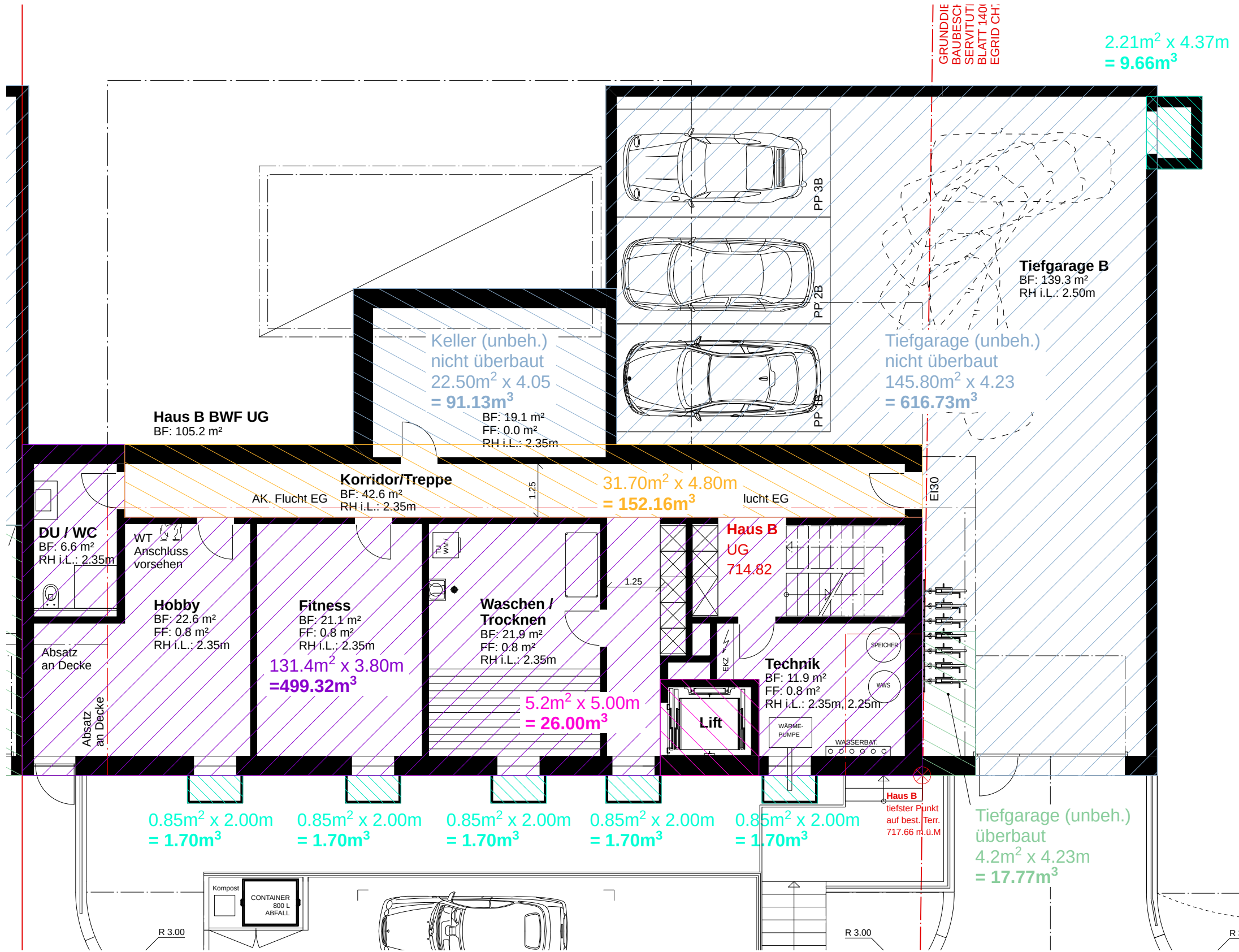
Untergeschoss
